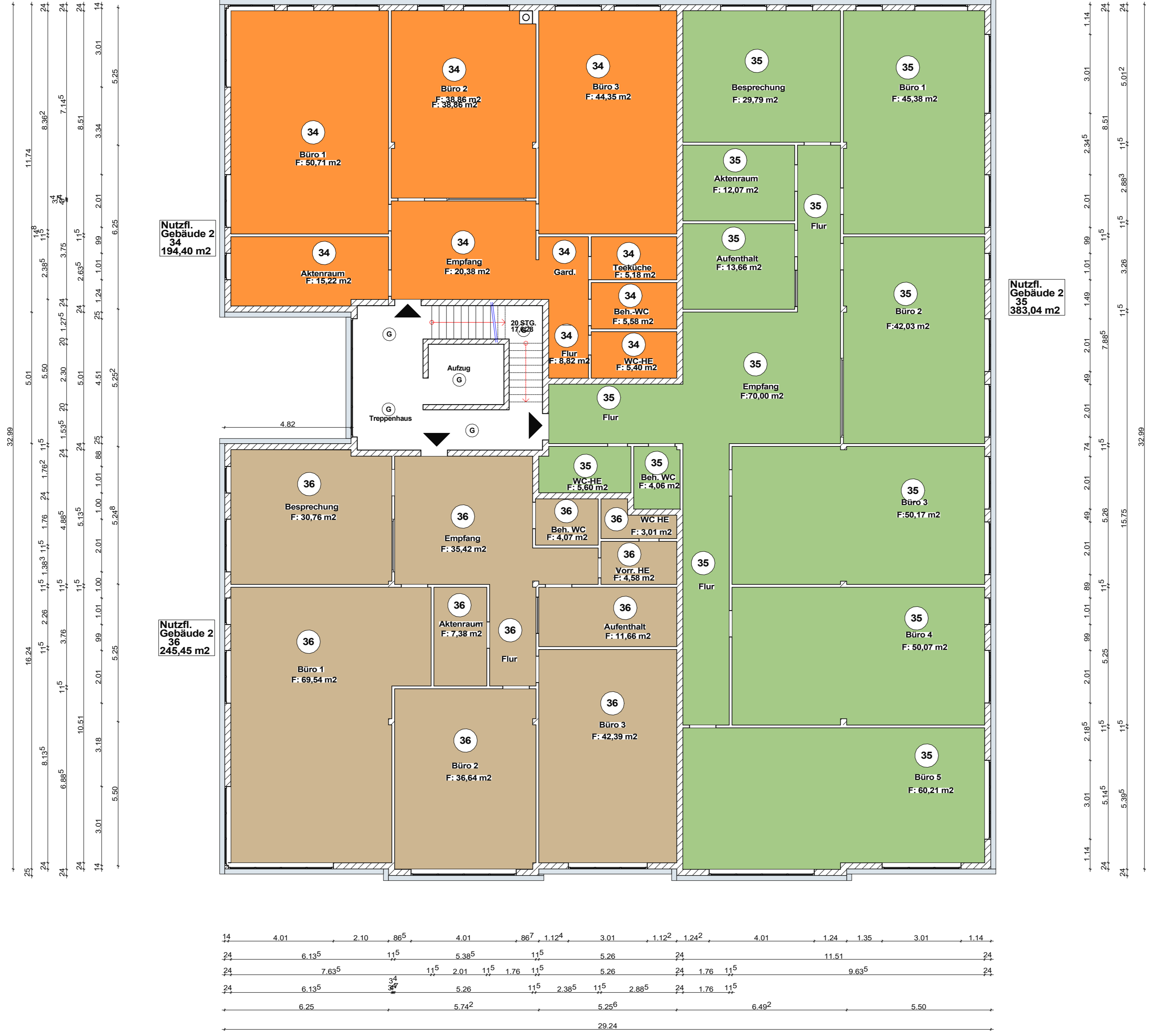
1. OBERGESCHOSS Gebäude 2
